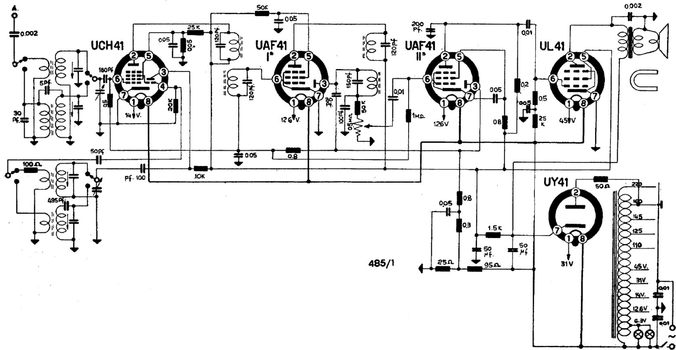
MINERVA RADIO - Mod. 485.1 «MONVISO» - Gamma medie da 200 a 580 m, gamma corte da 19 a 52 m. Media frequenza 470 kc/s. Altoparlante magnetodinamico. Potenza d'uscita 2,5 W. Consumo 25 W. (Valvole rimlock serie 100 mA).
